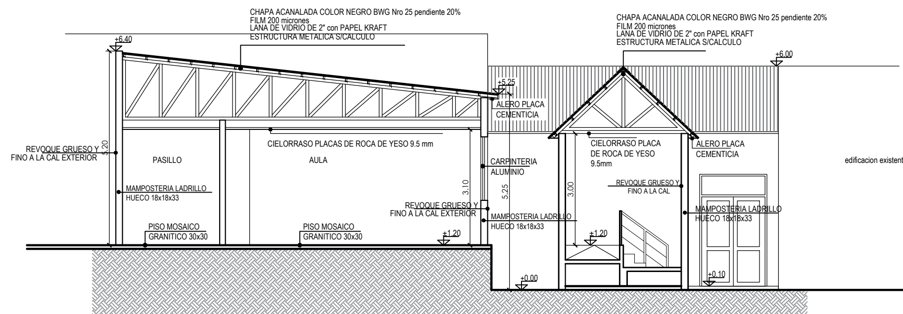
CORTE B-B
