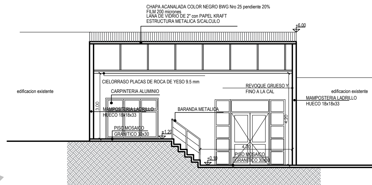
CORTE C-C
